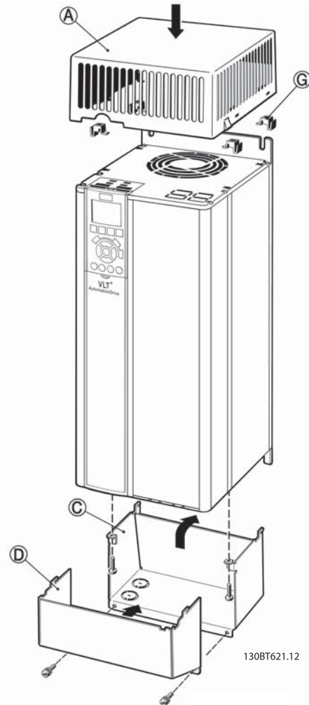
Behuizing B4, C3, C4 Eenheidsgrootte 24, 33, 34
