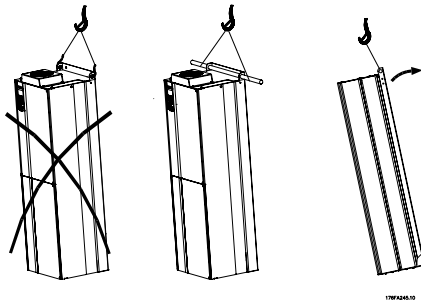
Afbeelding 5.3: Aanbevolen hijsmethode, framegrootte D en E .
