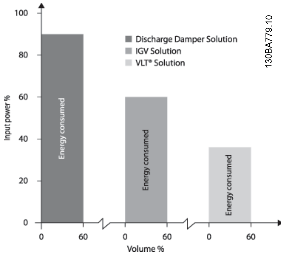
Afbeelding 2.7: Uitlaatkleppen verlagen het energieverbruik enigszins. Inlaatschoepen zorgen voor een besparing van 40% maar zijn duur om te installeren. De Danfoss frequentieomvormeroplossing verlaagt het energieverbruik met meer dan 50% en is eenvoudig te installeren.
