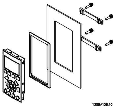
Afbeelding 3.5: LCP-set inclusief grafisch LCP, bevestigingsmateriaal, 3 m kabel en pakking
