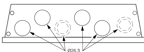
Afbeelding 5.9: Kabelinvoergaten voor behuizing A5. Het aangegeven gebruik van de gaten is enkel een aanbeveling; andere oplossingen zijn ook mogelijk.
