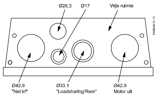
Afbeelding 5.12: Kabelinvoergaten voor behuizing B2. Het aangegeven gebruik van de gaten is enkel een aanbeveling; andere oplossingen zijn ook mogelijk.
