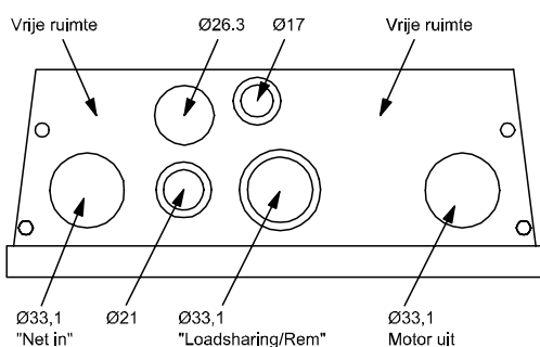
Afbeelding 5.10: Kabelinvoergaten voor behuizing B1. Het aangegeven gebruik van de gaten is enkel een aanbeveling; andere oplossingen zijn ook mogelijk.
