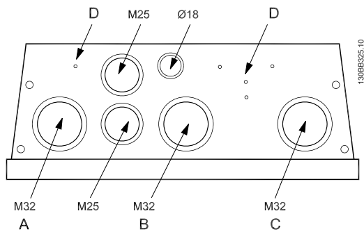
Afbeelding 5.11: Kabelinvoergaten voor behuizing B1. Het aangegeven gebruik van de gaten is enkel een aanbeveling; andere oplossingen zijn ook mogelijk.
