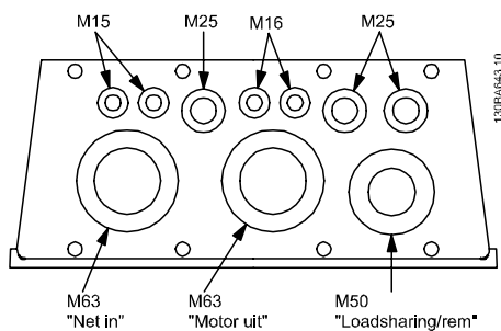
Afbeelding 5.14: Kabelinvoergaten voor behuizing C1. Het aangegeven gebruik van de gaten is enkel een aanbeveling; andere oplossingen zijn ook mogelijk.
