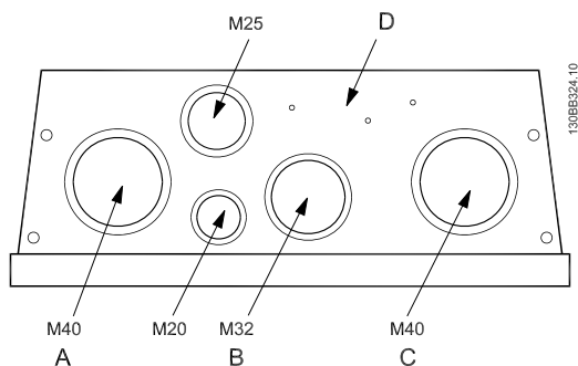
Afbeelding 5.13: Kabelinvoergaten voor behuizing B2. Het aangegeven gebruik van de gaten is enkel een aanbeveling; andere oplossingen zijn ook mogelijk.
