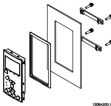
Afbeelding 3.6: LCP-set voor numeriek LCP, bevestigingsmateriaal en pakking
