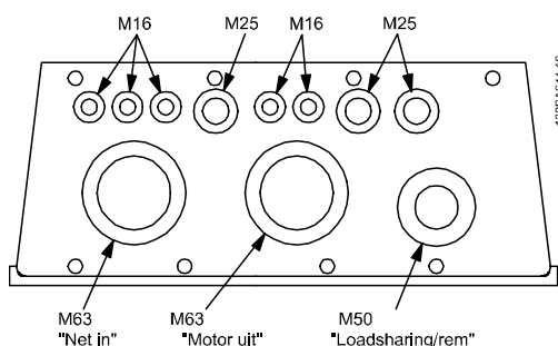
Afbeelding 5.15: Kabelinvoergaten voor behuizing C2. Het aangegeven gebruik van de gaten is enkel een aanbeveling; andere oplossingen zijn ook mogelijk.
