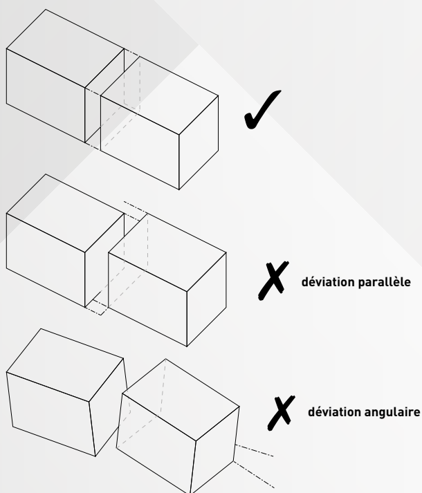
Figure 8 Alignement des composants
