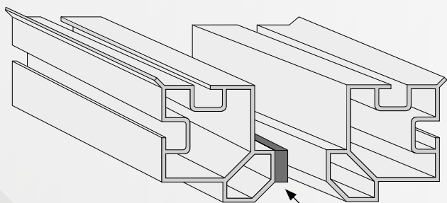
bande d'étanchéité en caoutchouc cellulaire 15 mm x 8 mm
