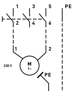
Figure 20 Raccordement de l'interrupteur de service Q1 en position 1-5-PE
