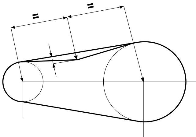
Figure 25 Profondeur d'indentation de la courroie
