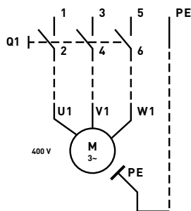
Figure 19 Raccordement de l'interrupteur de service Q1 en position 1-3-5-PE
