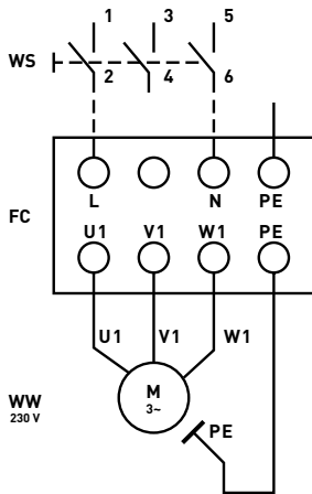
Figure 18 Raccordement de l'interrupteur de service WS en position 1-5-PE
