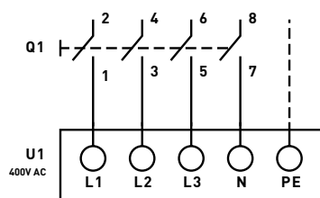
Figure 21 Raccordement de l'interrupteur de service Q1 en position 1-3-5-7-PE
