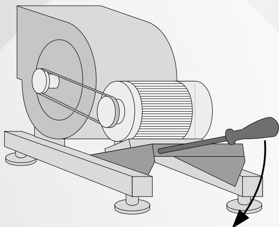
Figure 28 Tension à l'aide d'un tournevis
