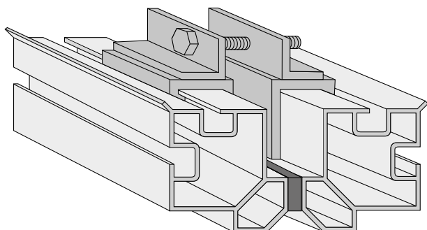
Figure 9 Raccords pour assembler les sections de la centrale
