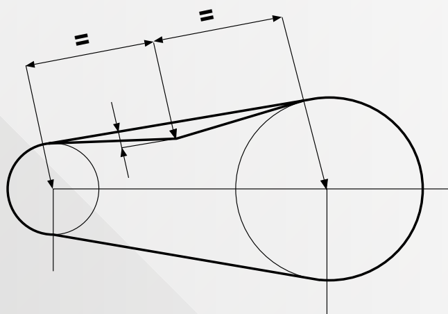
Figure 30 Profondeur d'indentation de la courroie
