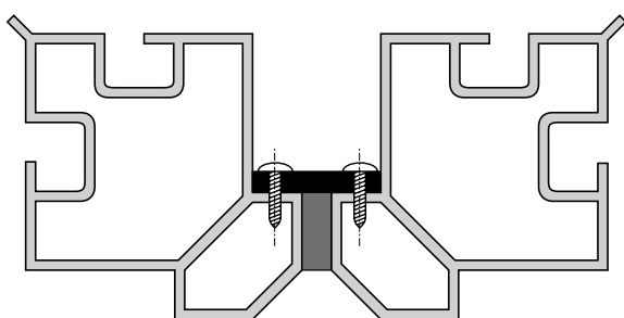
Figure 11 Raccords entre les sections de la centrale
