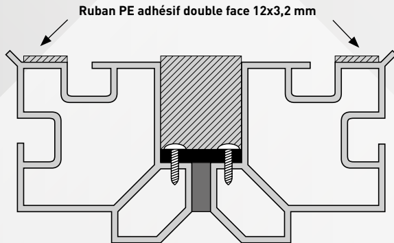
Figure 13 Isoler la jonction
