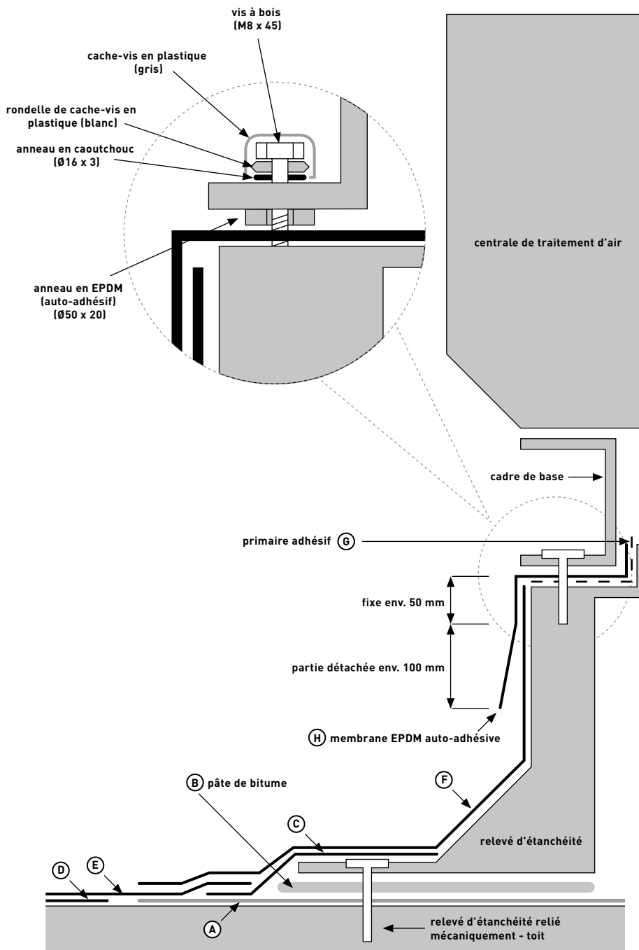
Figure 5 illustration détaillée du relevé d'étanchéité
