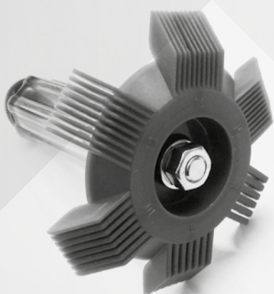
Figure 23 Peigne à lamelles
