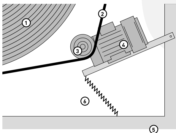
Figure 22a Roue thermique et moteur
