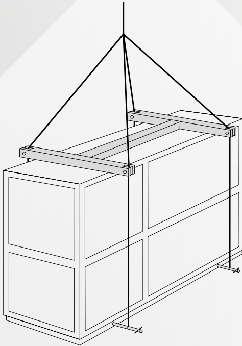
Figure 3 Utilisez une entretoise entre les 2 balanciers.
