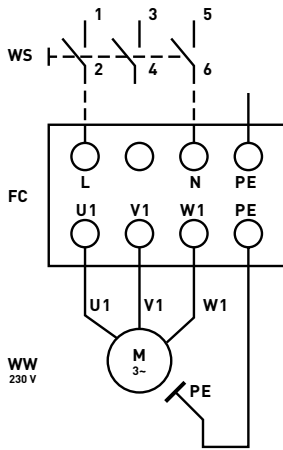
Abbildung 18 Betriebsschalter WS in Stellung 1-5-PE anschließen
